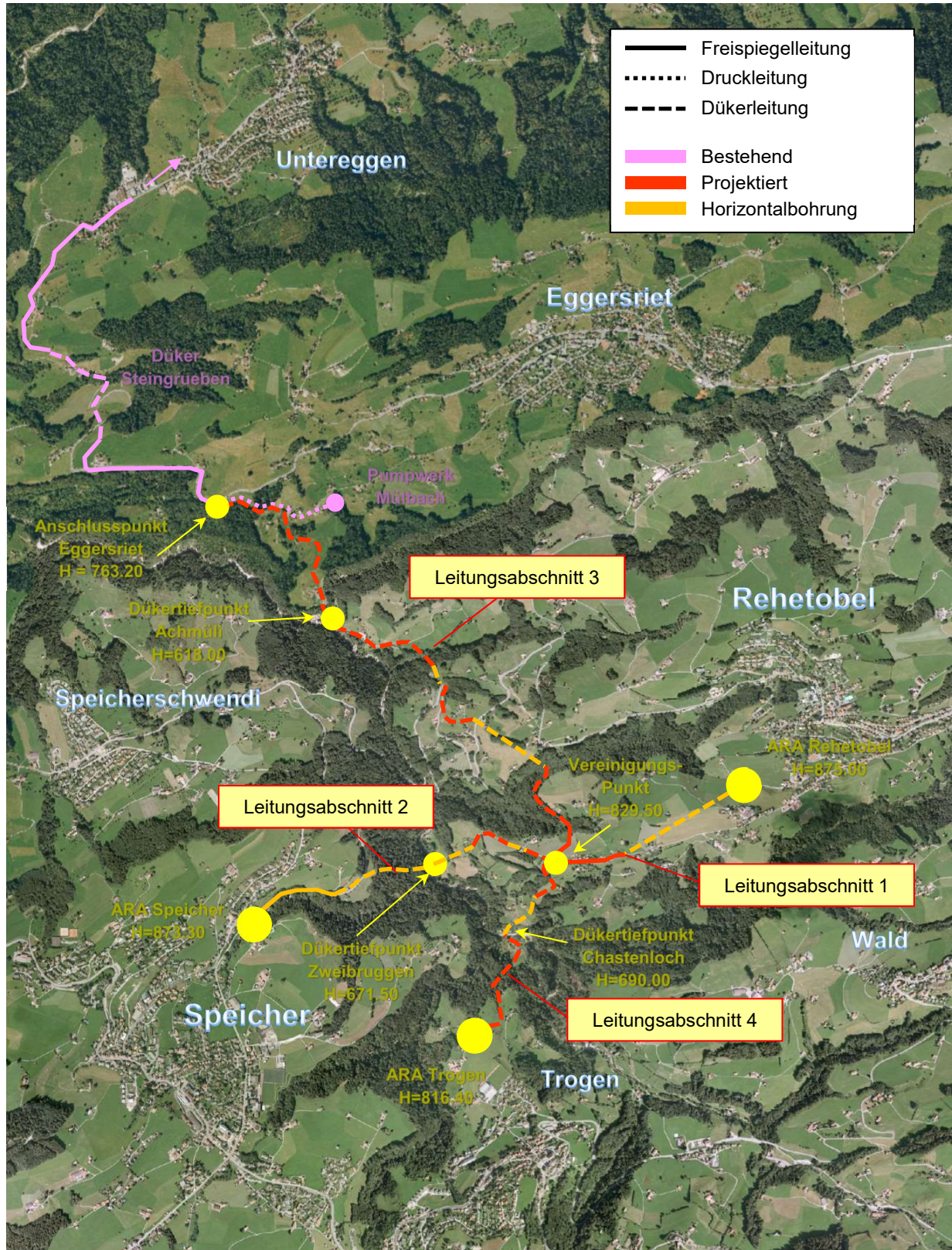
Situationsplan Anschluss ARA Trogen-Wald an Anschlusspunkt/ Vereinigungspunkt bei der Lobenschwendi in Rehetobel
